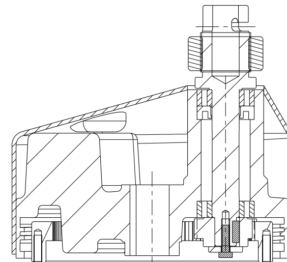
SEZIONE A-A
